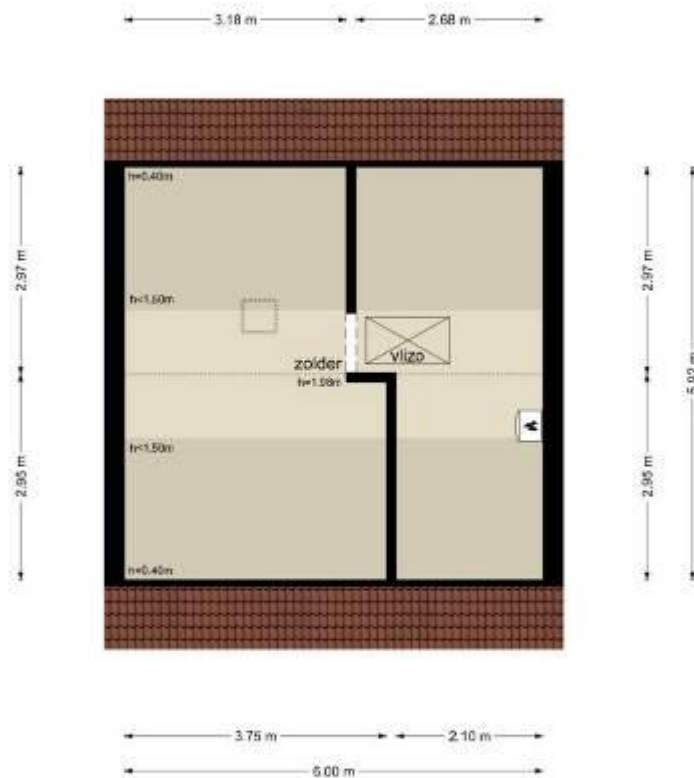
Zuivelstraat 14 - Didam Tweede Verdieping
